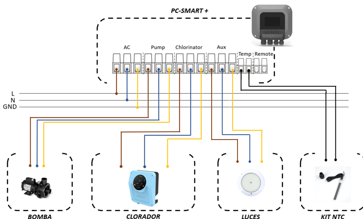
Fig. 3: Ejemplo de conexionado básico.
