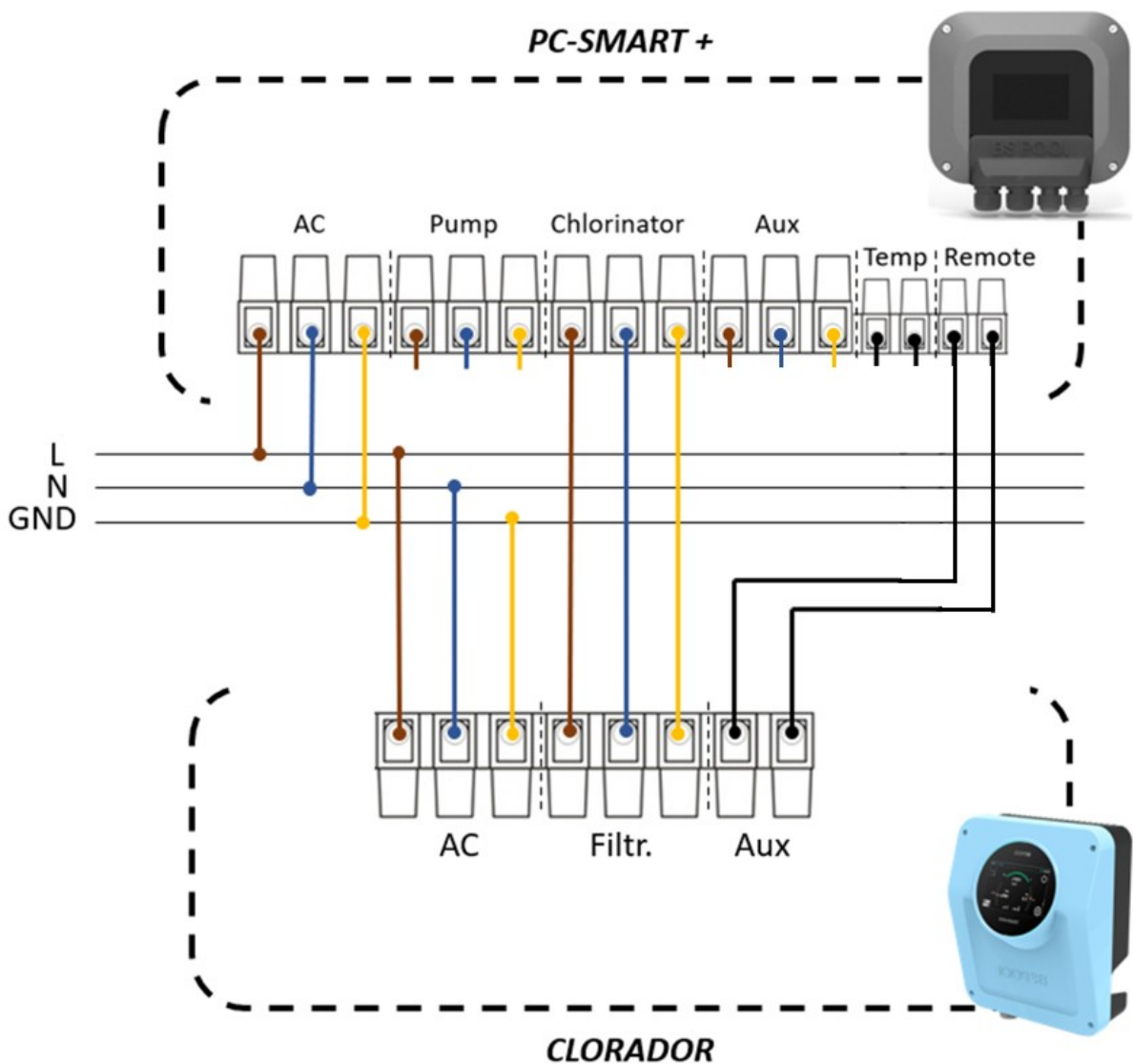
Fig. 4: Ejemplo de conexionado Remoto.
